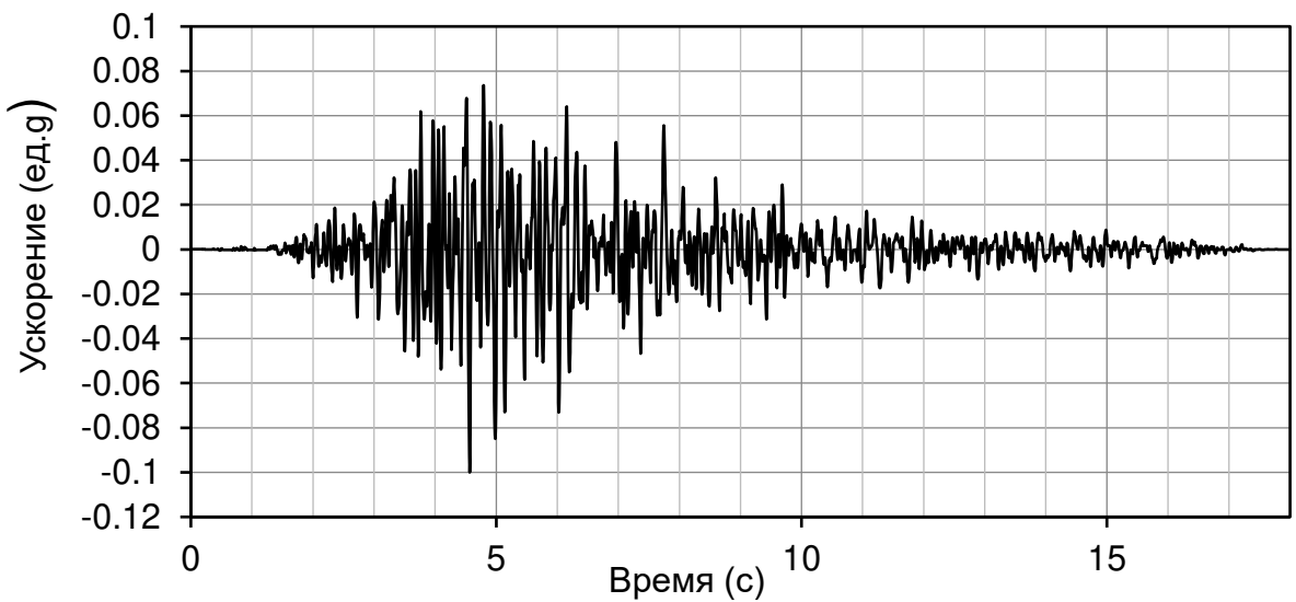
Рисунок 5.4.2 – Синтезированная акселерограмма для нижней отметки толщи инженерно-геологического разреза; ускорение указано в единицах ускорения свободного падения g
