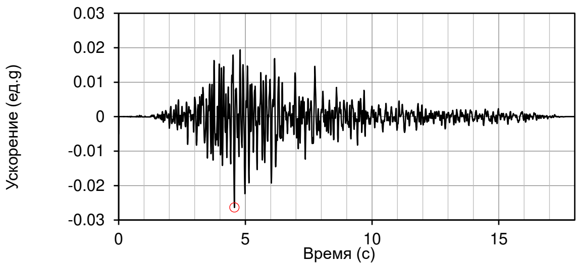
Рисунок 5.4.1 – Горизонтальная компонента акселерограммы землетрясения Umbria Marche (aftershock 4); ускорение указано в единицах ускорения свободного падения g
