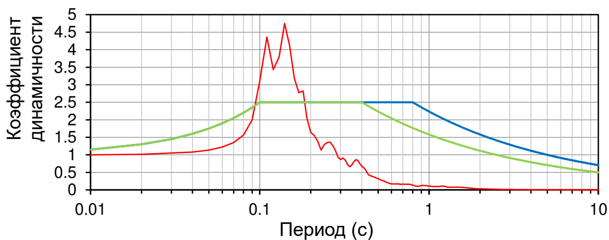
Рисунок 5.4.6 – Спектр коэффициентов динамичности акселерограммы для верхней границы грунта; зеленая кривая соответствует нормативному спектру
