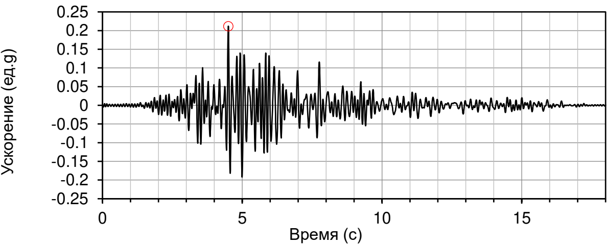
Рисунок 5.4.3 – Рассчитанная акселерограмма для верхней границы грунта; ускорение указано в единицах ускорения свободного падения g .
