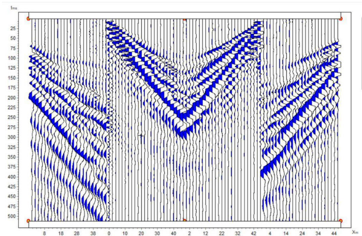
Рисунок 5.3.2 – Визуализация сейсмограм СЗ-2. Р-Волны
