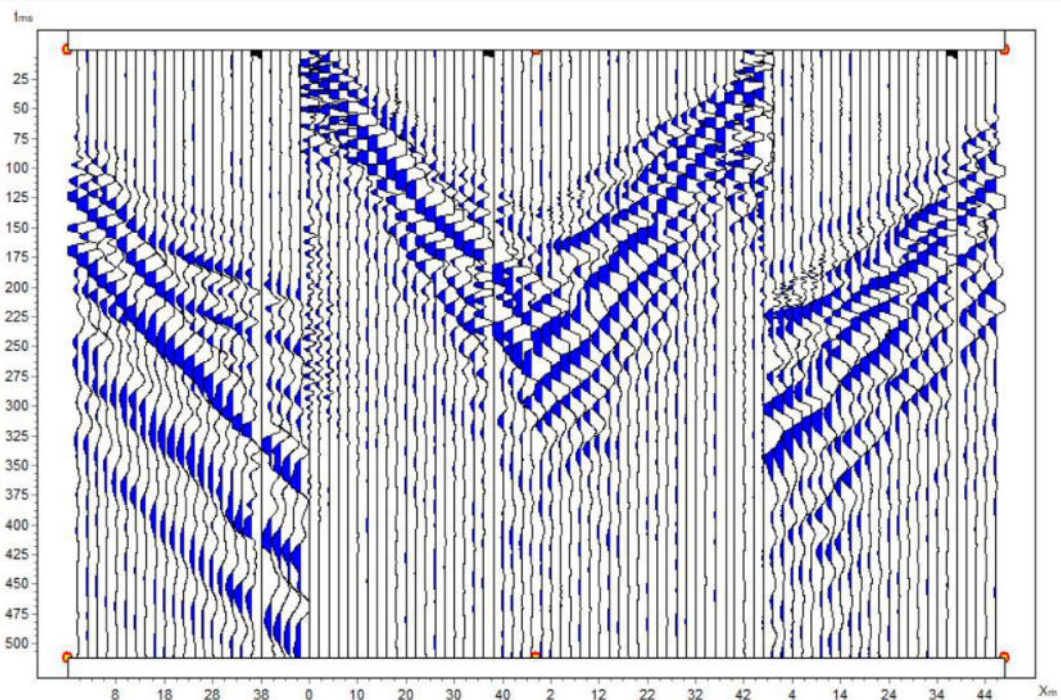
Рисунок 5.3.3 – Визуализация сейсмограм С3-2. S-волны
