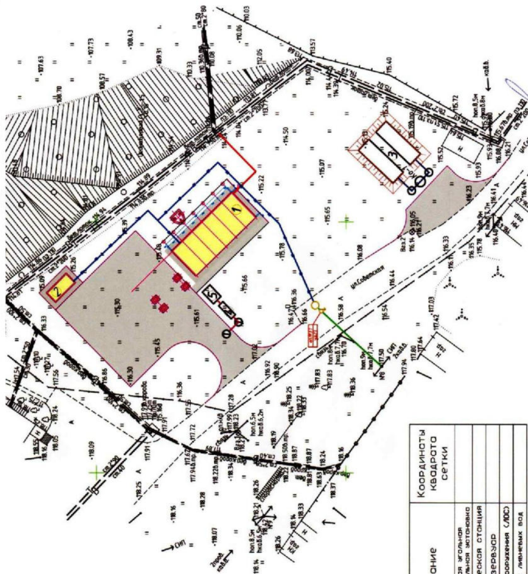
Приложение 2. План проектируемых зданий и сооружений
