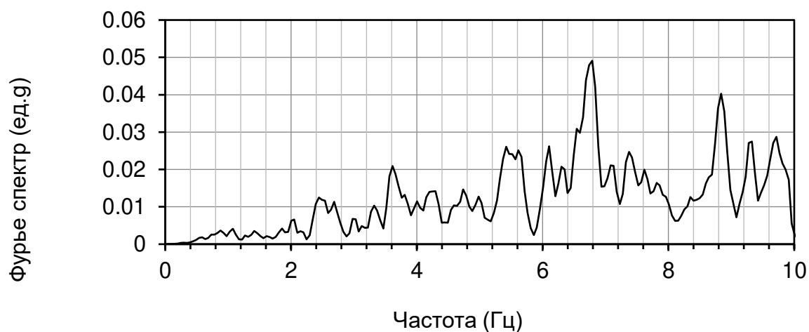
Рисунок 5.4.4 – Фурье спектр акселерограммы для верхней границы грунта
