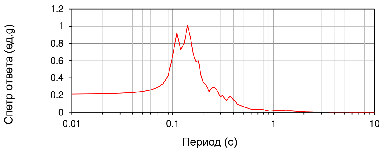
Рисунок 5.4.5 – Спектр ответа акселерограммы для верхней границы грунта в единицах ускорения свободного падения g
