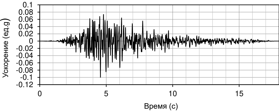
Рисунок 5.4.2 – Синтезированная акселерограмма для нижней отметки толщи инженерно-геологического разреза; ускорение указано в единицах ускорения свободного падения g
