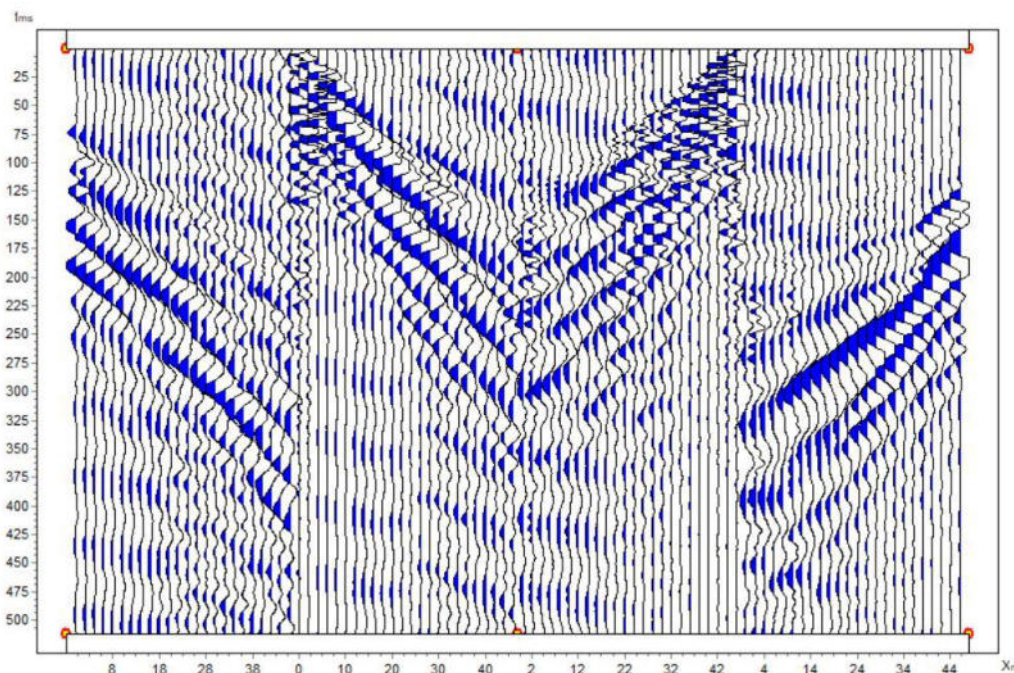
Рисунок 5.3.3 – Визуализация сейсмограм СЗ-2. S-волны
