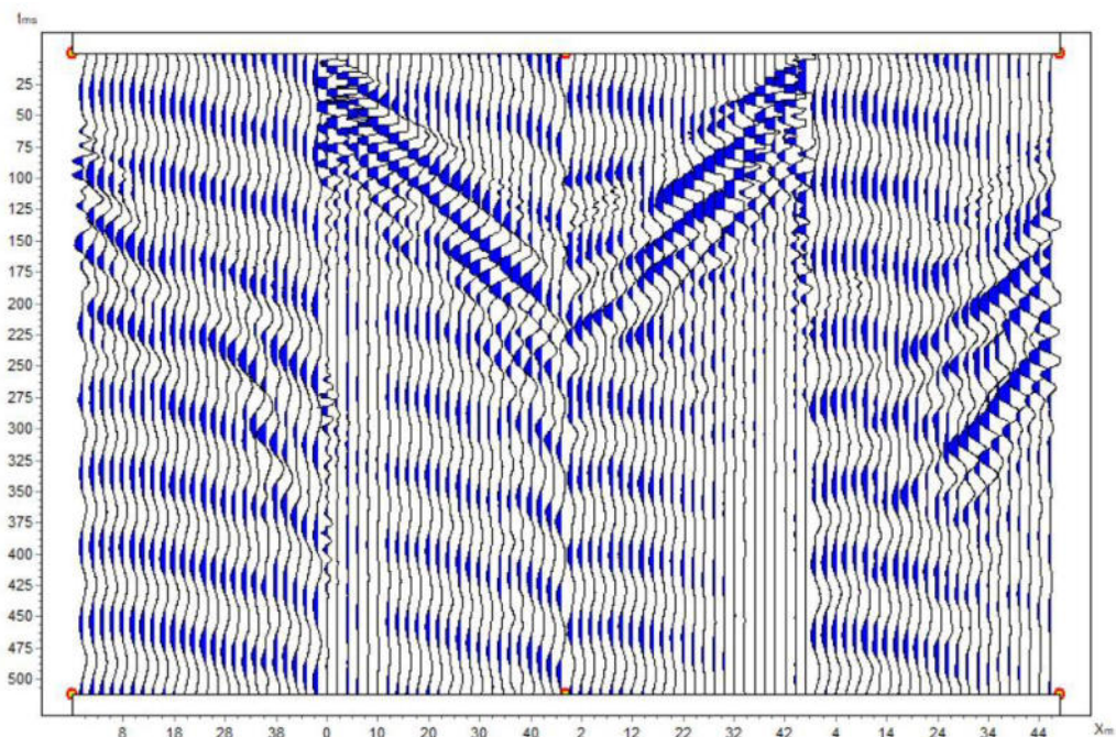
Рисунок 5.3.2 – Визуализация сейсмограм СЗ-2. Р-Волны
