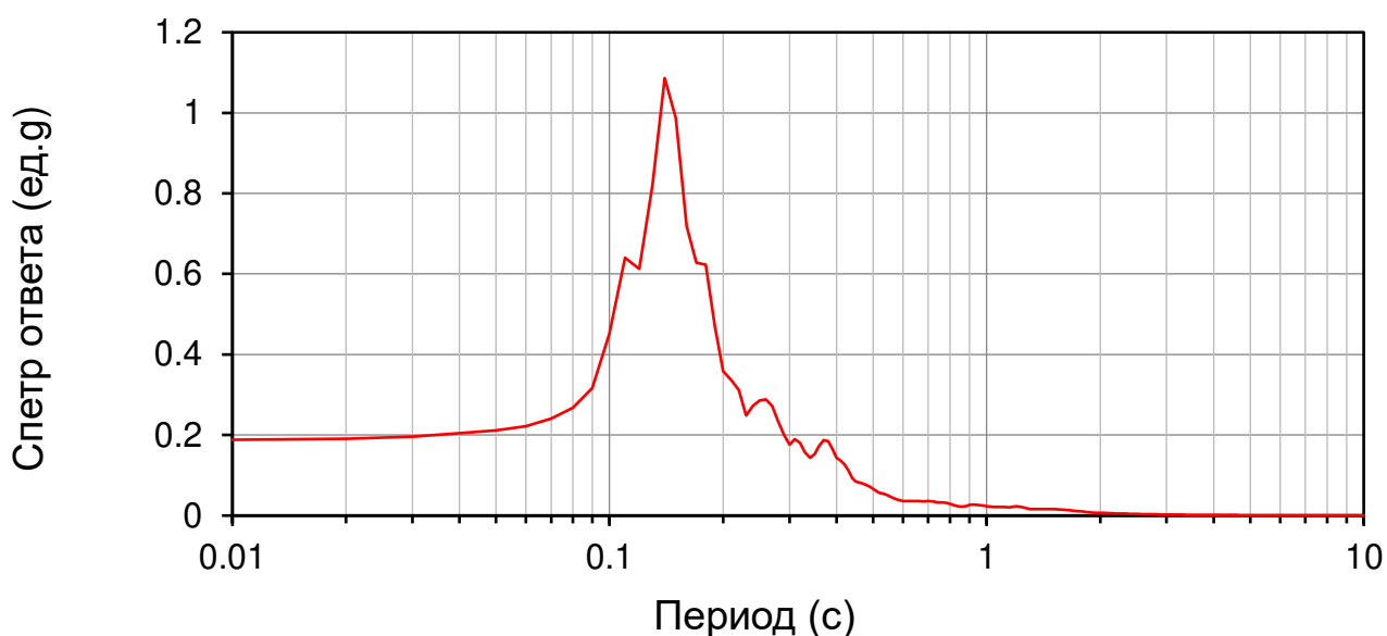
Рисунок 5.4.5 – Спектр ответа акселерограммы для верхней границы грунта в единицах ускорения свободного падения g
