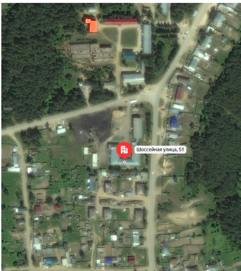
Рисунок 1 – Площадка изысканий
