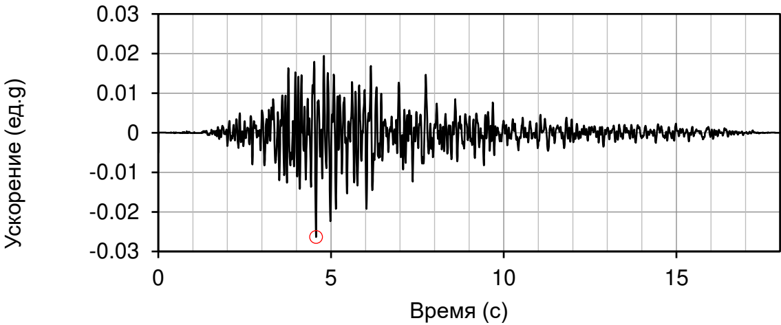
Рисунок 5.4.1 – Горизонтальная компонента акселерограммы землетрясения Umbria Marche (aftershock 4); ускорение указано в единицах ускорения свободного падения g
