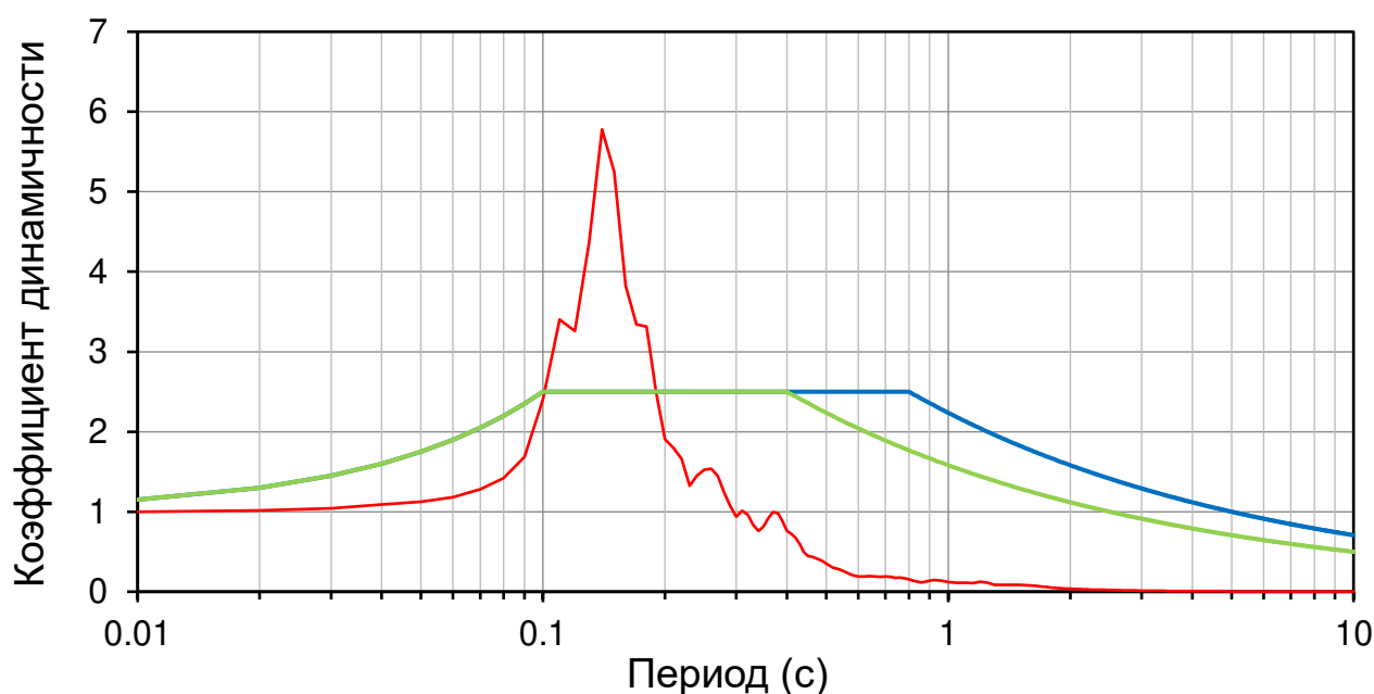
Рисунок 5.4.6 – Спектр коэффициентов динамичности акселерограммы для верхней границы грунта; зеленая кривая соответствует нормативному спектру коэффициентов динамичности для грунтов I и II категории по СНиП II-7-81*, а синяя – для грунтов III категории и IV категории.
