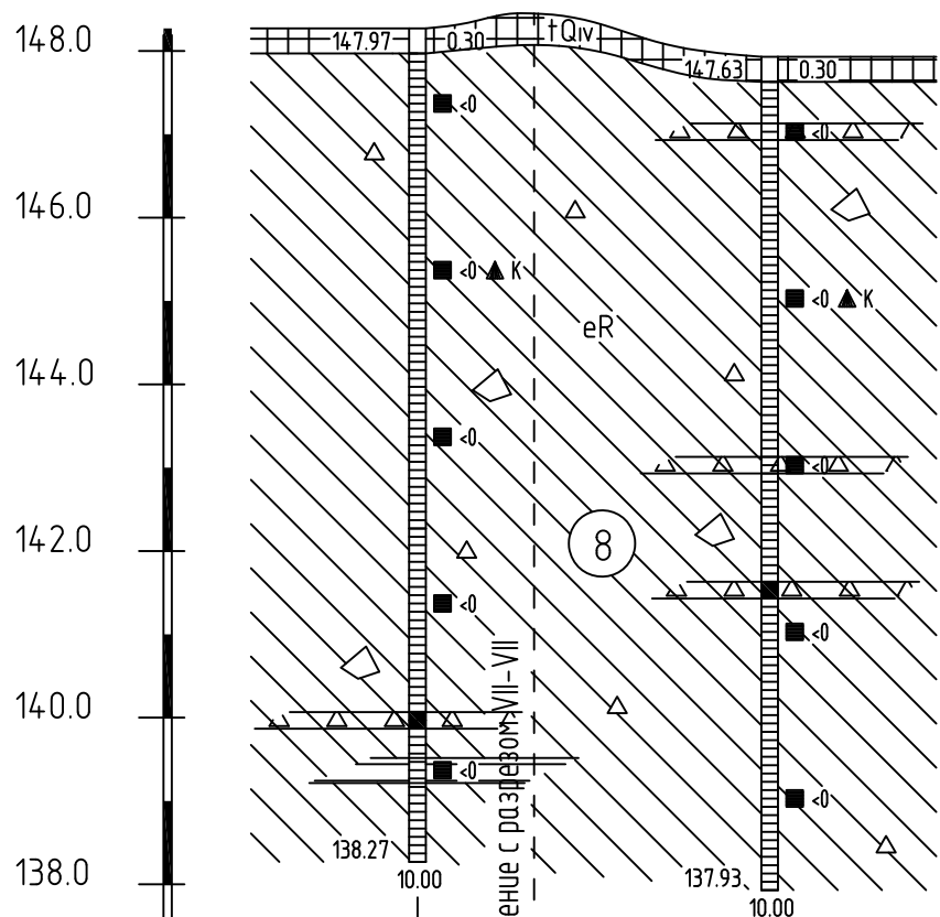
Инженерно-геологический разрез по линии I-I
