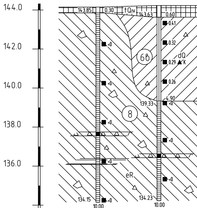
Инженерно-геологический разрез по линии III-III
