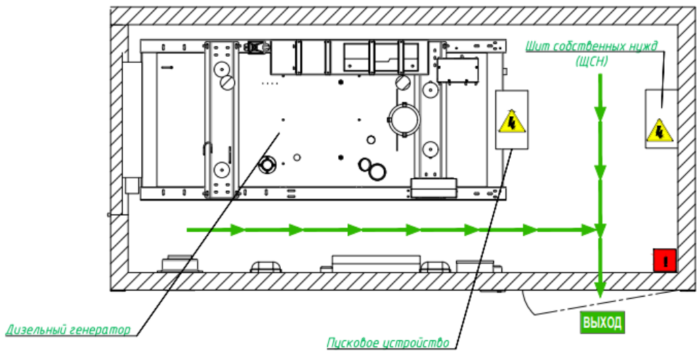
Схема эвакуации
