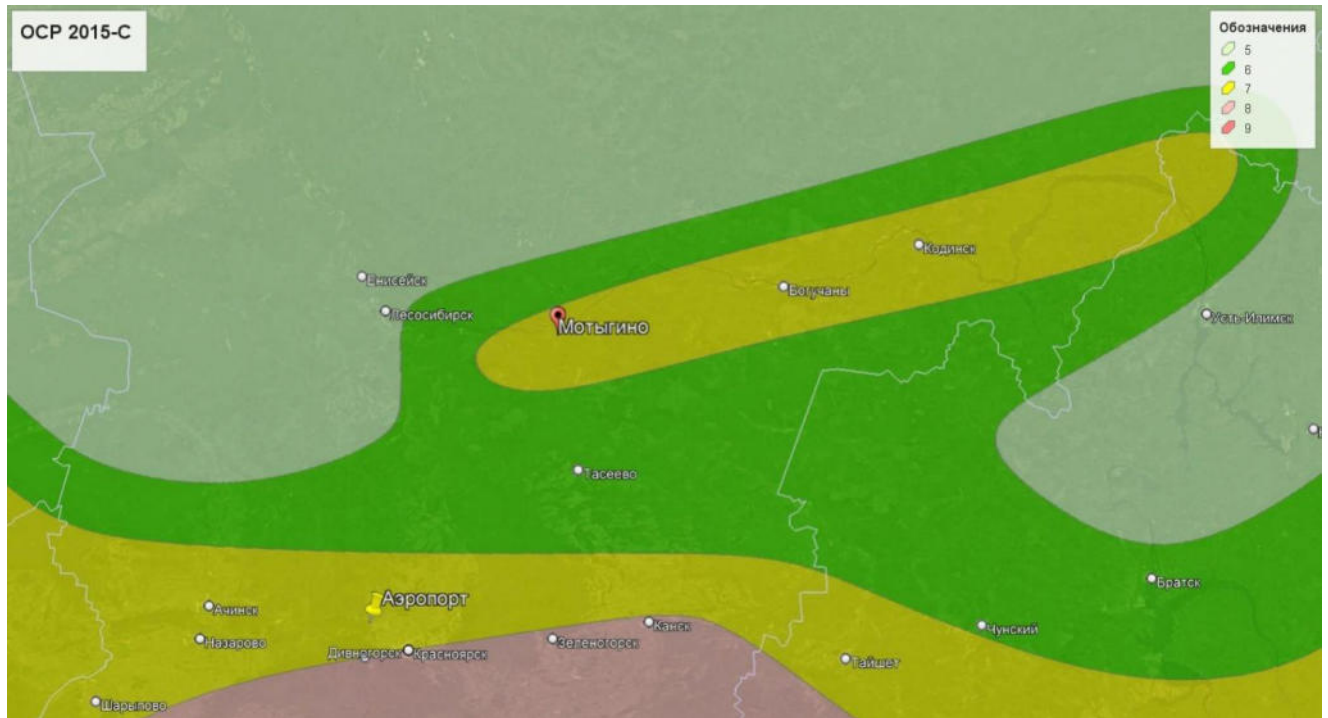
Рисунок 5.1.1 – Фрагменты карт общего сейсмического районирования ОСР-2015
