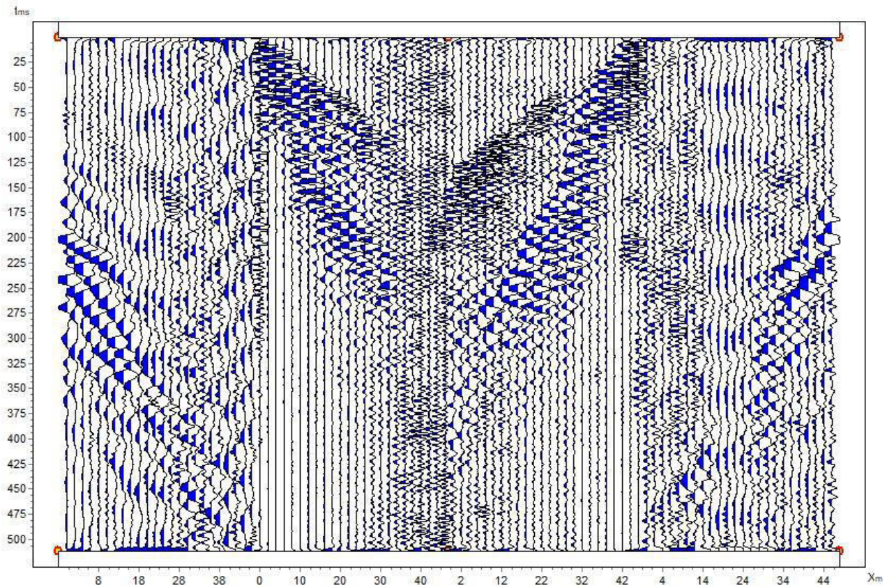
Рисунок 5.3.3 – Визуализация сейсмограм СЗ-2. S-волны
