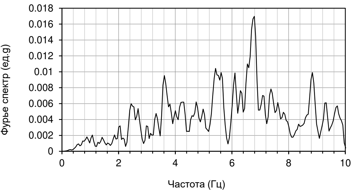
Рисунок 5.4.4 – Фурье спектр акселерограммы для верхней границы грунта
