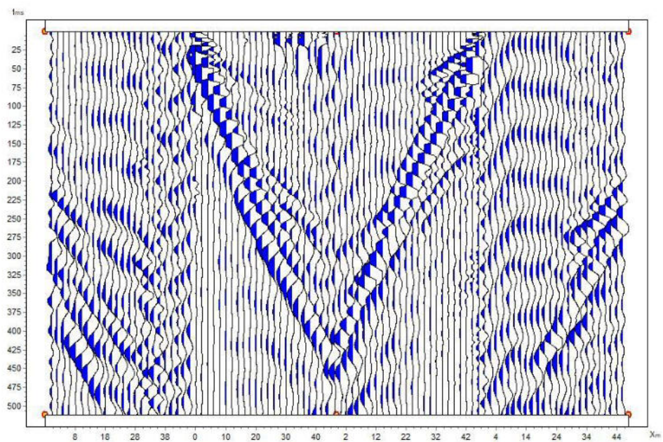
Рисунок 5.3.2 – Визуализация сейсмограм СЗ-2. Р-Волны
