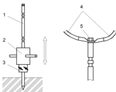
Рис 2. Приспособление для забивки стержней заземления
