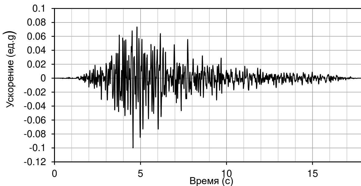
Рисунок 5.4.2 – Синтезированная акселерограмма для нижней отметки толщи инженерно-геологического разреза; ускорение указано в единицах ускорения свободного падения g
