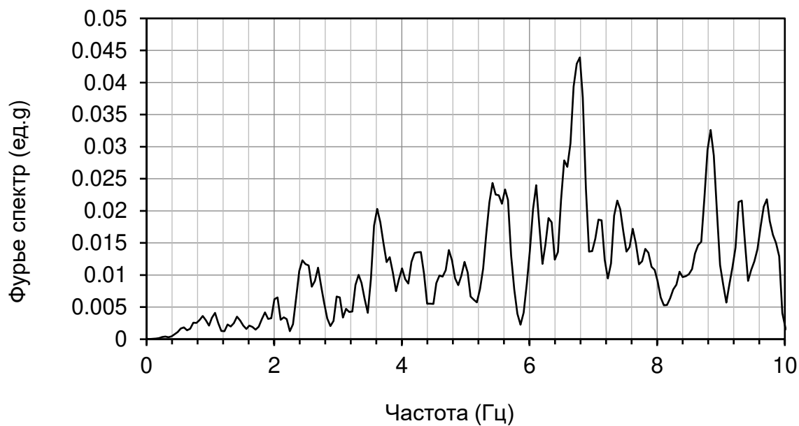
Рисунок 5.4.4 – Фурье спектр акселерограммы для верхней границы грунта
