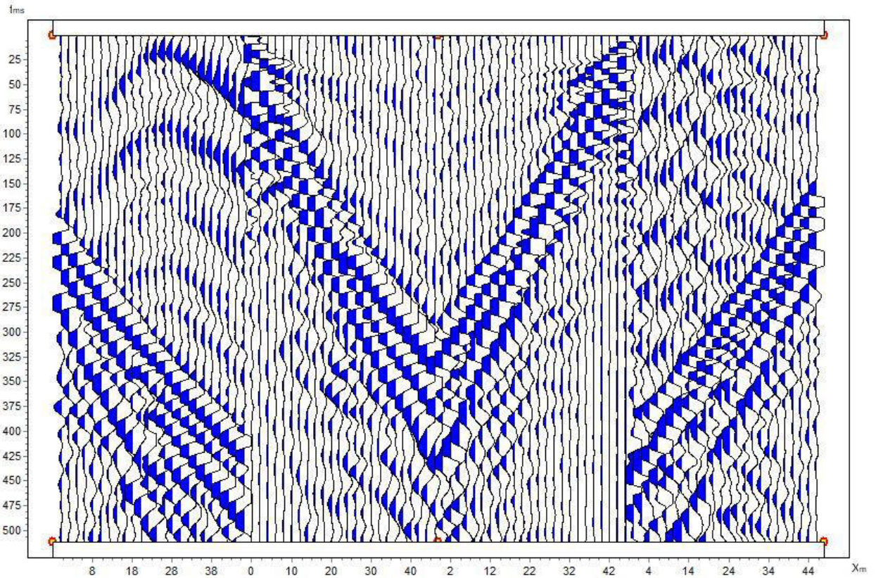
Рисунок 5.3.2 – Визуализация сейсмограм СЗ-2. Р-Волны
