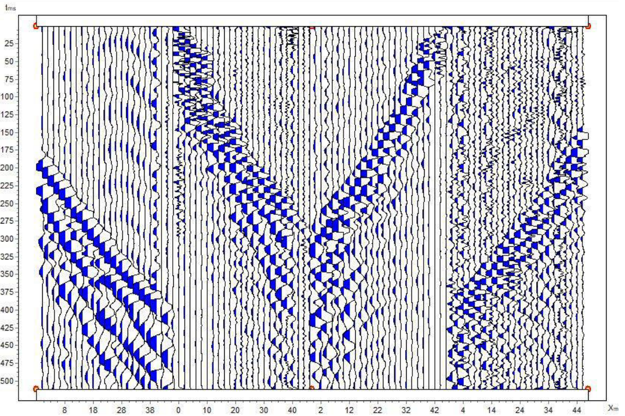
Рисунок 5.3.3 – Визуализация сейсмограм СЗ-2. S-волны
