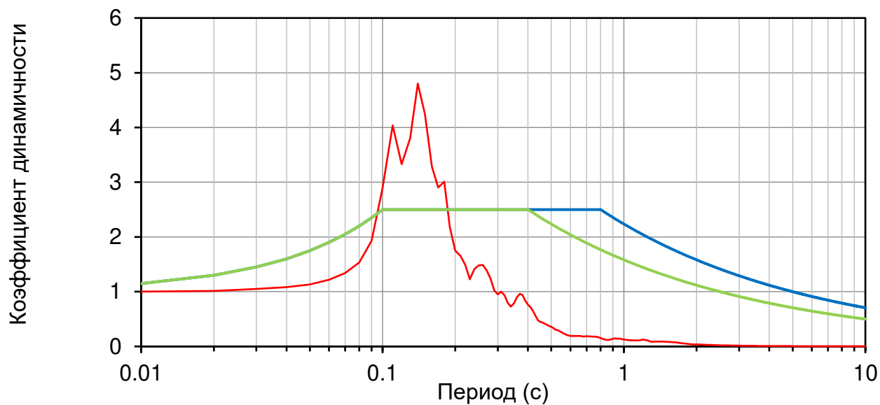
Рисунок 5.4.6 – Спектр коэффициентов динамичности акселерограммы для верхней границы грунта; зеленая кривая соответствует нормативному спектру коэффициентов динамичности для грунтов I и II категории по СНиП II-7-81*, а синяя – для грунтов III категории и IV категории.
