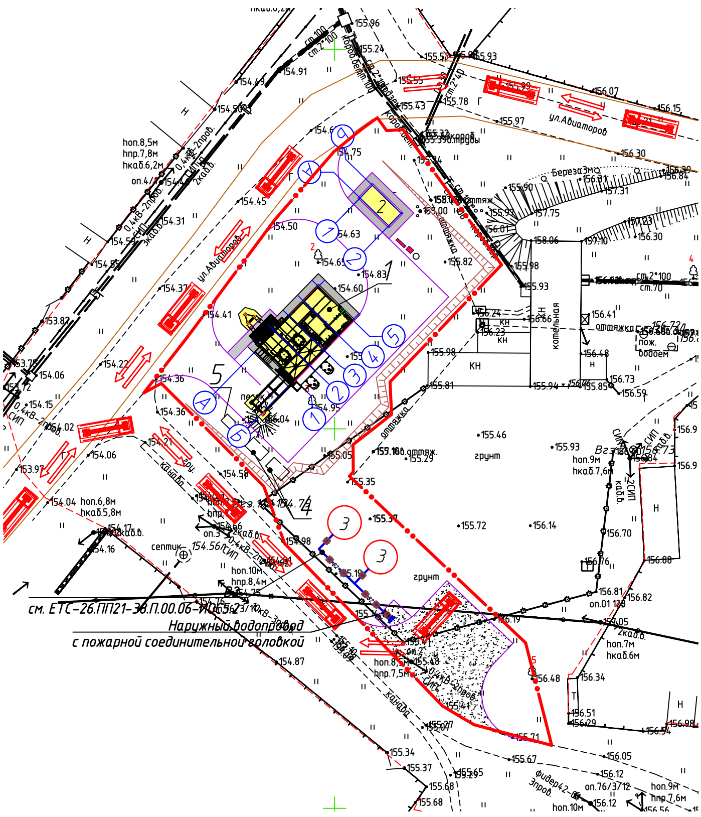
Схема пожарного проезда
