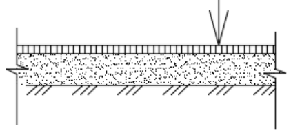
Рисунок 1 – Конструкция восстанавливаемого асфальтобетонного покрытия тротуара
