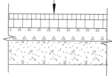
Рисунок 2 - Конструкция восстанавливаемого асфальтобетонного покрытия проезда
