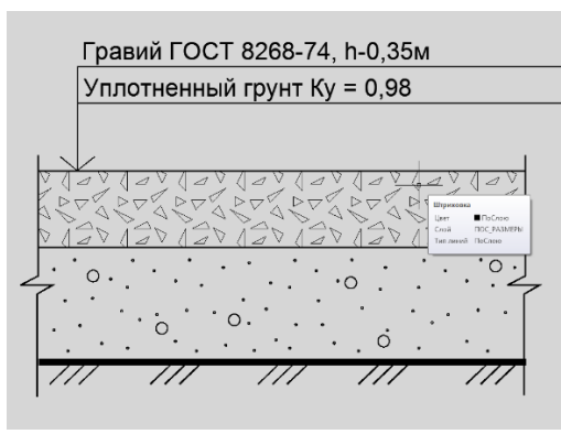
Рисунок 3 - Конструкция восстанавливаемого гравийного покрытия проезда
