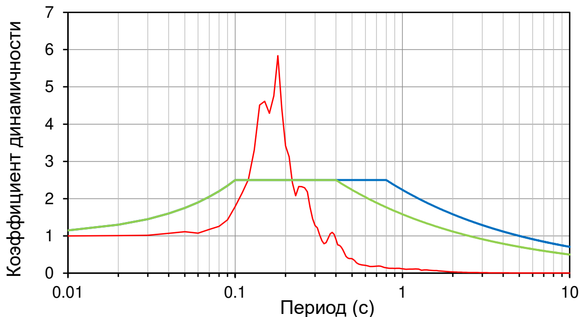
Рисунок 5.4.6 – Спектр коэффициентов динамичности акселерограммы для верхней границы грунта; зеленая кривая соответствует нормативному спектру коэффициентов динамичности для грунтов I и II категории по СНиП II-7-81*, а синяя – для грунтов III категории и IV категории.
